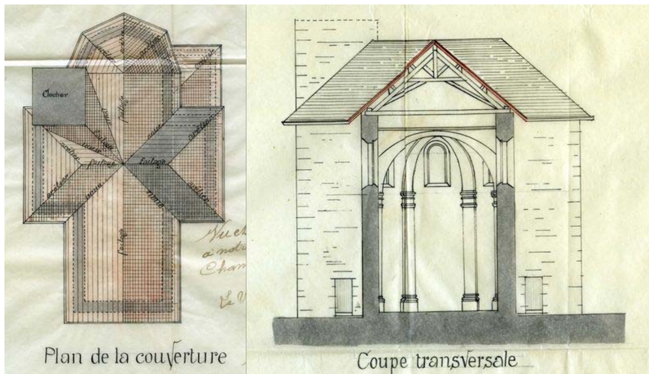
Plan de l'église pour les travaux de grosses réparations de 1897 (235 E-dépôt 187)
