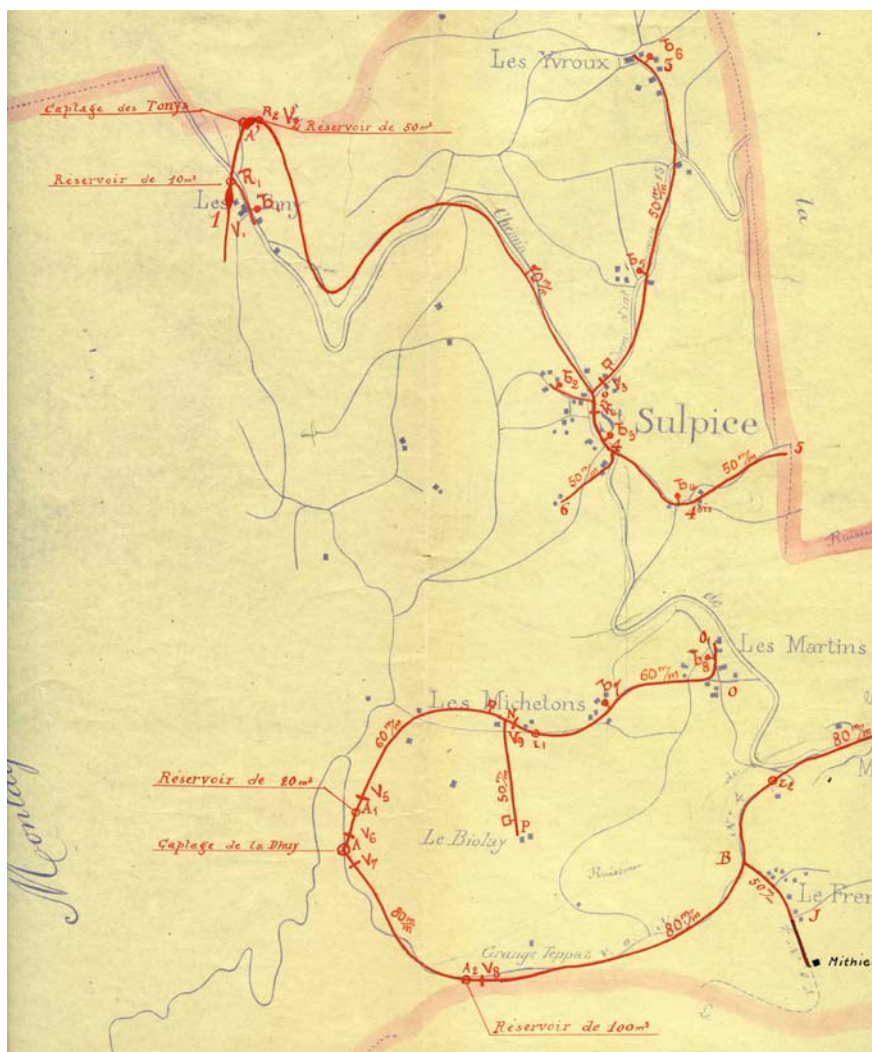
Extrait d'un projet de plan de réseau d'eau potable de 1933 (235 E-dépôt 212)
